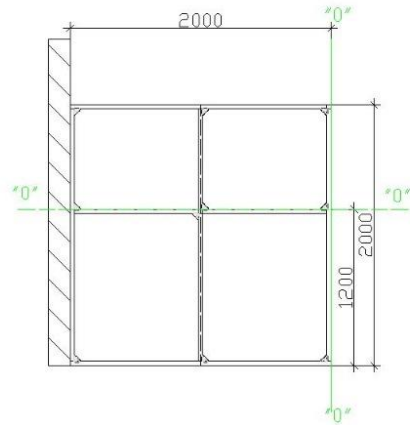
Вид слева
